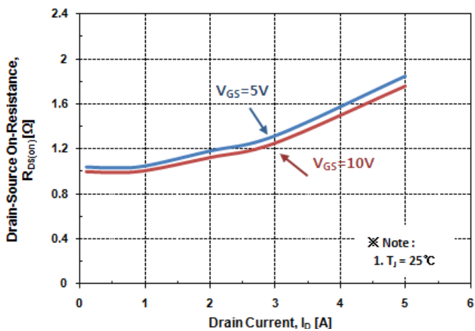
Fig. 3 R_{DS(ON)} - I_D
