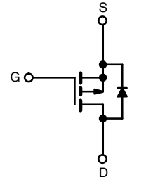
P-Channel MOSFET
