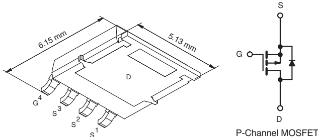
P-Channel MOSFET
